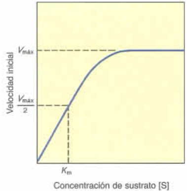
Fig. 2-34. Diagrama de la velocidad de reacción de una enzima a concentraciones de sustrato cada vez mayores. En el texto se describen la V_{m\acute{a}x} y la K_m . La curva es una hipérbola cuya primera parte sigue una cinética de primer orden (es decir, la reacción es proporcional a la concentración del sustrato); la segunda parte corresponde a la saturación, que tiene una cinética de orden cero (ya que no depende de la concentración del sustrato).
