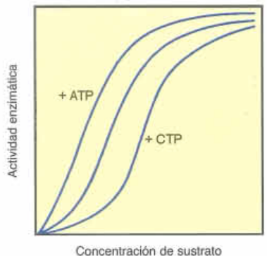
Fig. 2-35. Cinética de la enzima alostérica ATPasa, que muestra una curva sigmoidea característica en lugar de una hipérbola. Obsérvense los efectos de un activador (ATP) y de un inhibidor (CTP).
